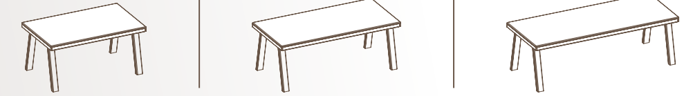
DU.TA160 FIX/T 160 x 98 x 78 cm DU.TA200 FIX/T 200 x 98 x 78 cm DU.TA240 FIX/T 240 x 98 x 78 cm
